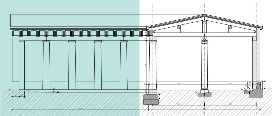
↓ Αποκατάσταση της ανατολικής στοάς του Αρτεμείου της Αμαρύνθου (τα σωζόμενα κατάλοιπα αποδίδονται με γκρι σκούρο χρώμα). Reconstruction of the eastern portico of the Artemision at Amarnthos (preserved remains in dark grey).
