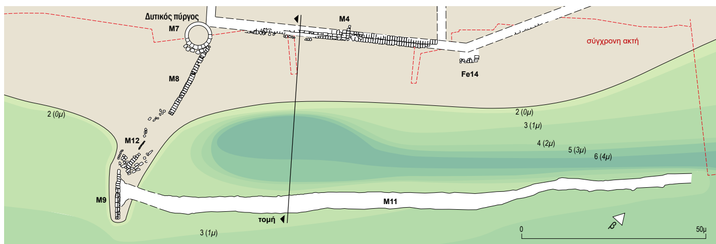
Κάτοψη και τομή της δυτικής λιμενικής λεκάνης. Plan and section of the western harbour basin.
